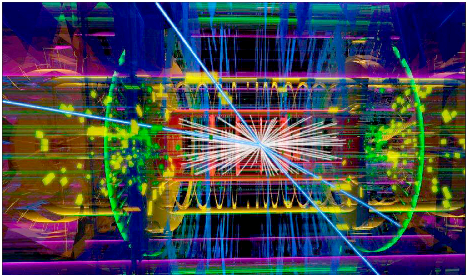
HIGGS-BOSONETS FØDSEL: En av kollisjonene fra ATLAS-eksperimentet der det ser ut til å ha bli lagd et Higgs-boson. De blå/hvite linjene kommer ut fra midten av bildet og viser hvor fire myoner som man regner med kom fra Higgs-bosonet tok veien. ILLUSTRASJON: ATLAS EXPERIMENT © 2012 CERN
