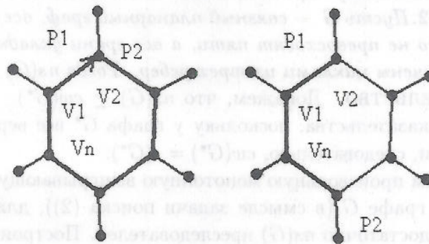
Рис. 2. К доказательству теоремы 1.
