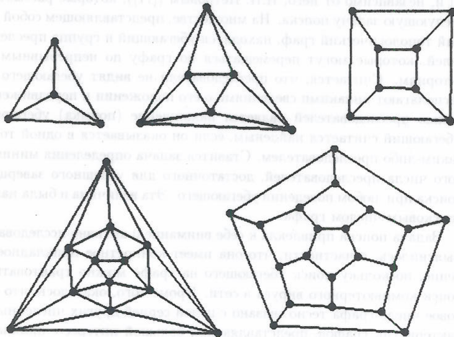
Рис. 1. Графы правильных многогранников: тетраэдра, октаэдра, куба, икосаэдра, додекаэдра.
